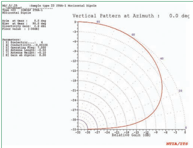
Fig.7. Dipolo ubicado a un décimo de longitud de onda del suelo
