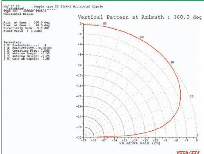
Fig.6. Dipolo ubicado a un cuarto de longitud de onda del suelo
