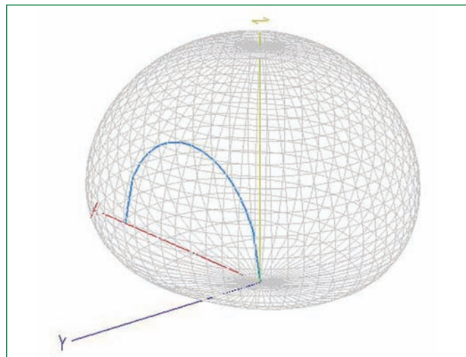
Fig.9. Diagrama de radiación de una antena NVIS de medio bucle
